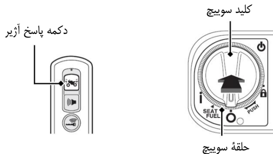
حلقه سویچ
