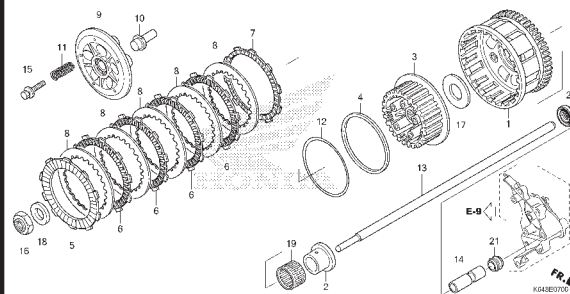
E-7 CLUTCH
