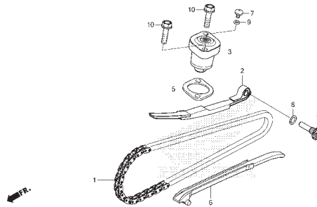
E-5 CAM CHAIN/TENSIONER
